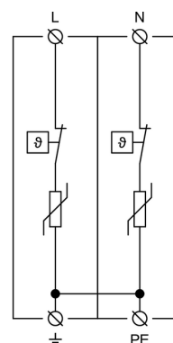
Vnútrotná schéma zapojenia
